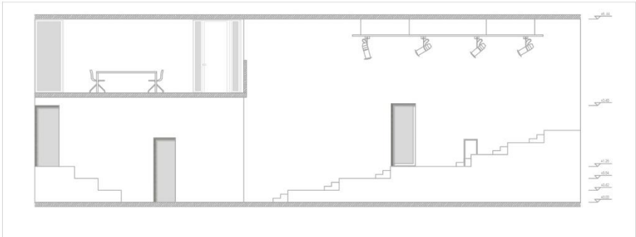
ELEVATION B-B
